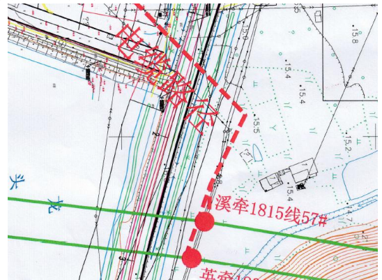
图 1-3 电缆穿越北湖西街
