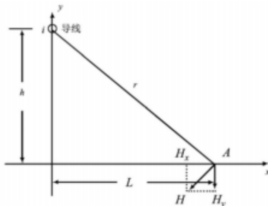
图 4 磁场向量图
