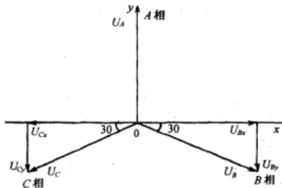
图 1 对地电压计算图
