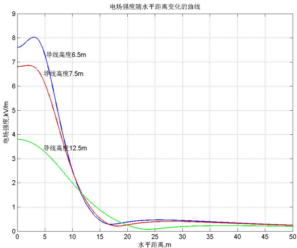
图 A-1 220kV 双回架空线路电场强度随水平距离变化趋势图
