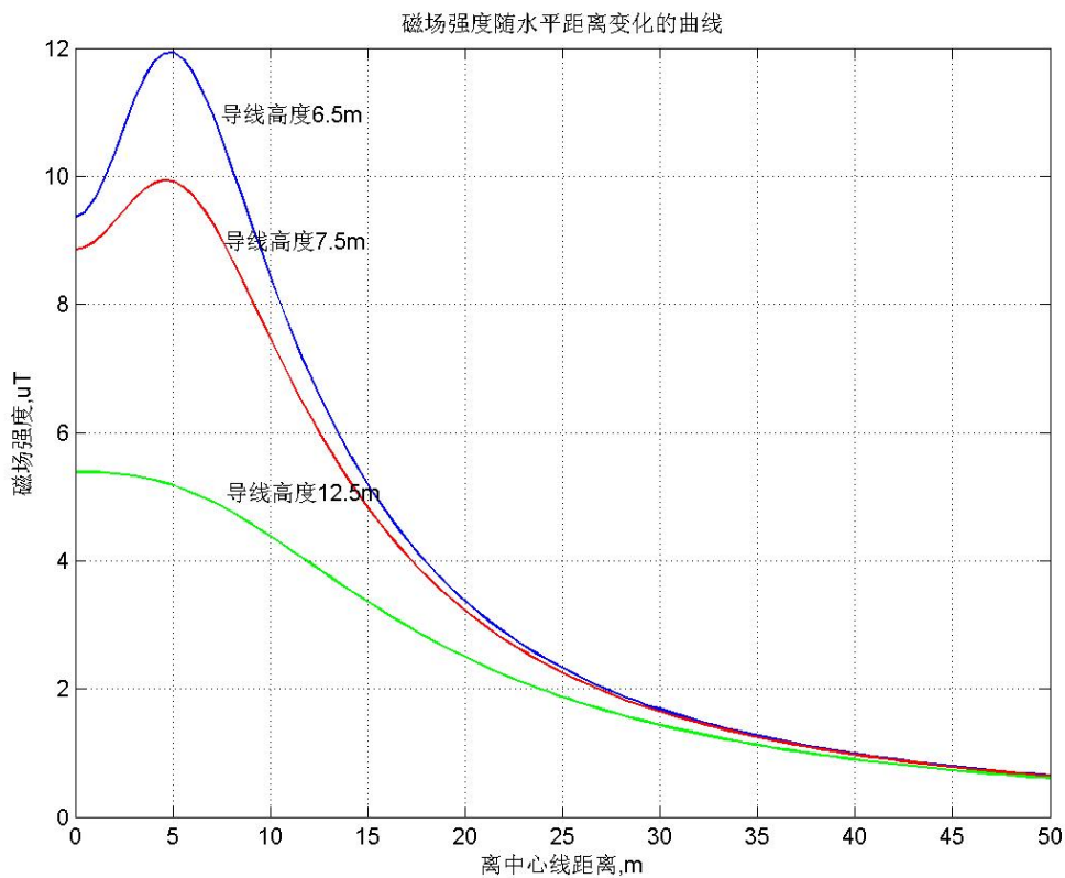
图 A-2 220kV 双回架空线路磁场强度随水平距离变化趋势图
