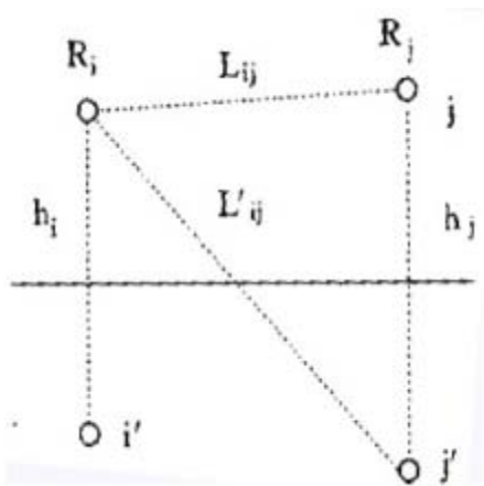
图 2 电位系数计算图
