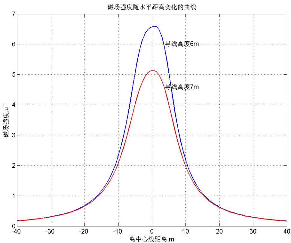
图 A-6 110kV 单回架空线路磁场强度随水平距离变化趋势图
