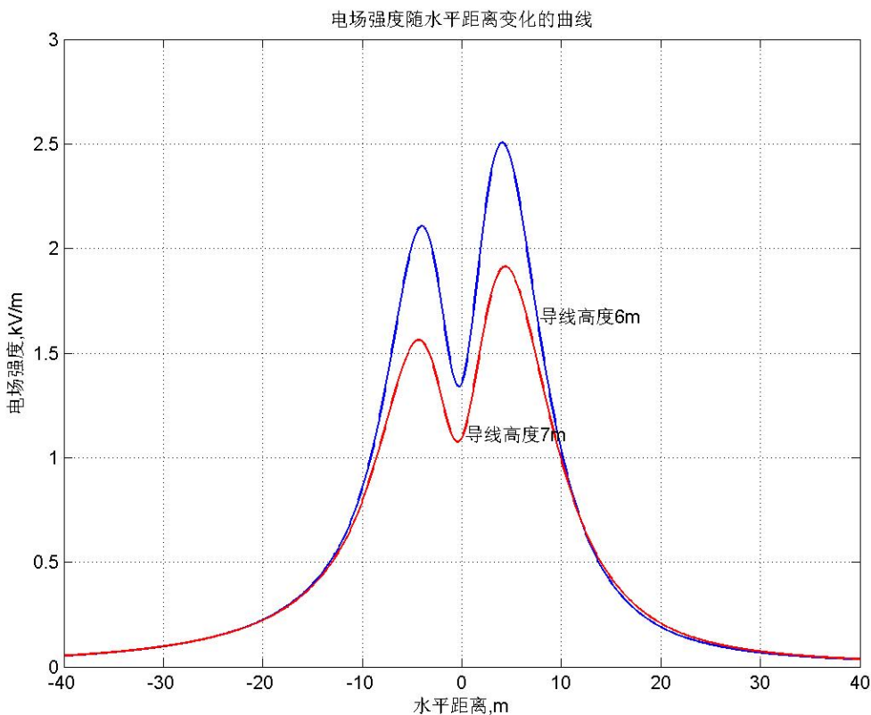
图 A-5 110kV 单回架空线路电场强度随水平距离变化趋势图
