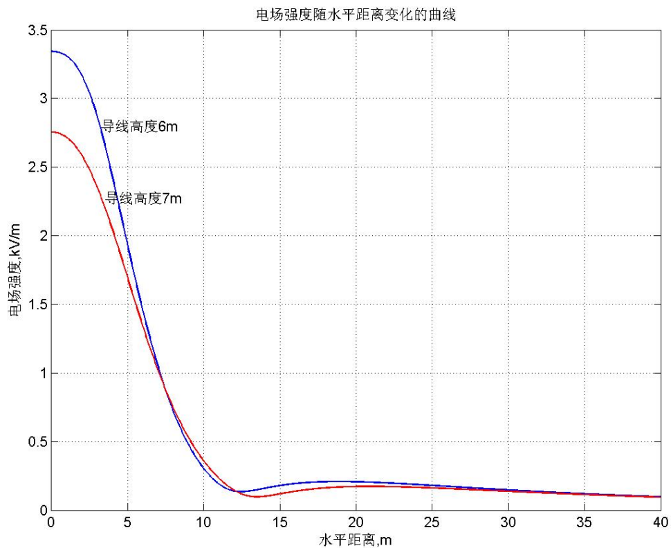
图 A-3 110kV 双回架空线路电场强度随水平距离变化趋势图
