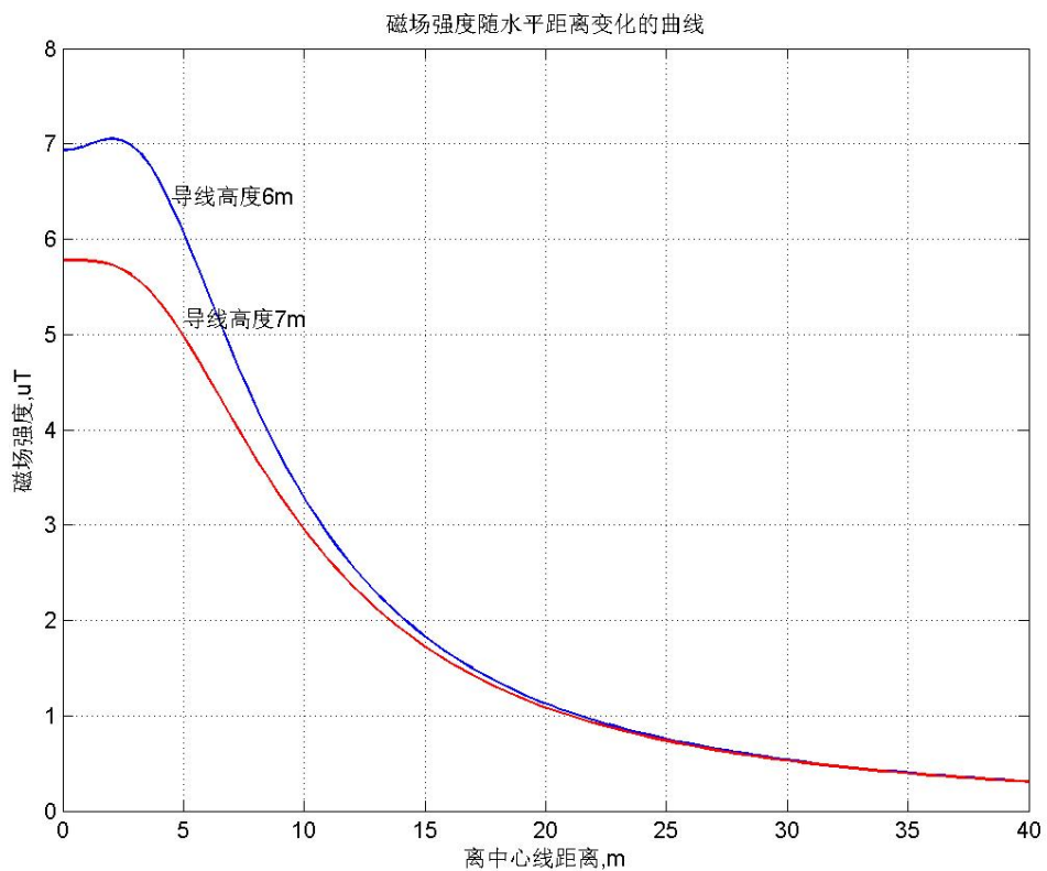
图 A-4 110kV 双回架空线路磁场强度随水平距离变化趋势图
