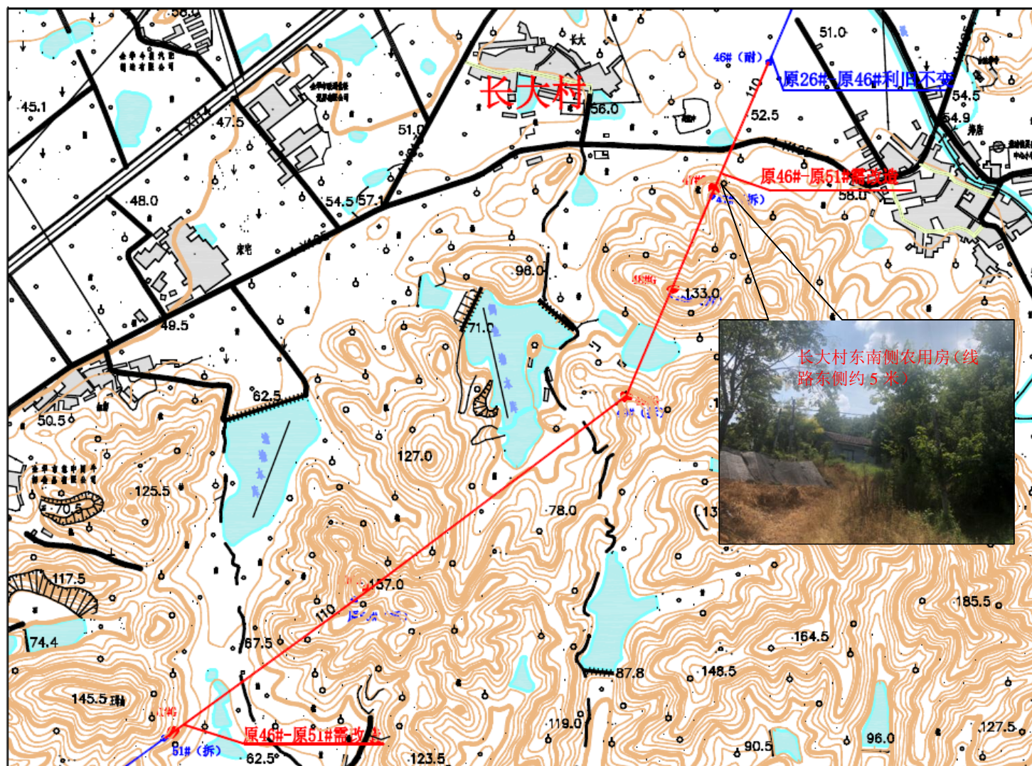
附图 2-2 线路路径图
