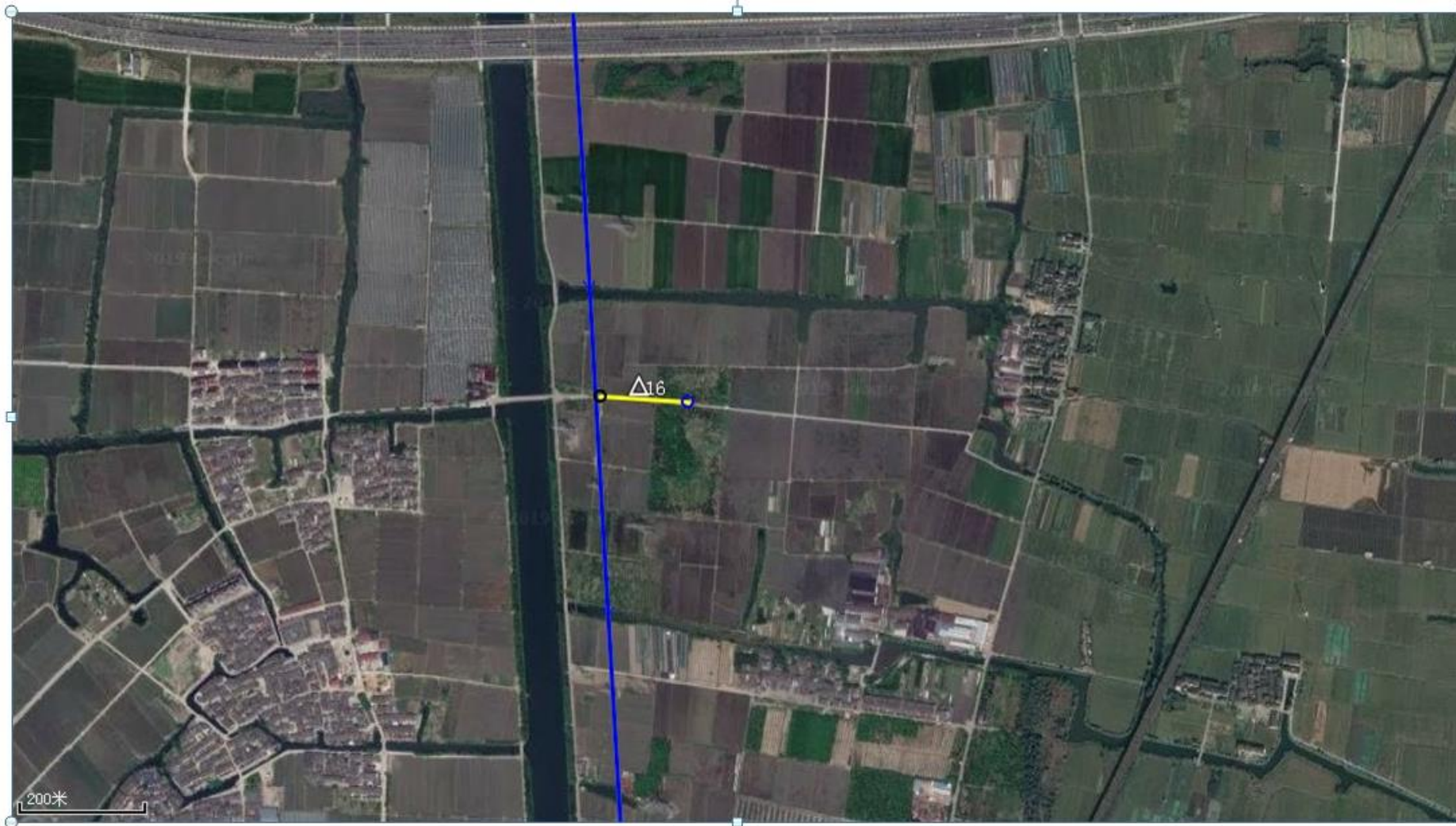
附图 3-3 (k) 220kV 天一~芦江输电线路工程 ▲ 16 检测点位示意图
