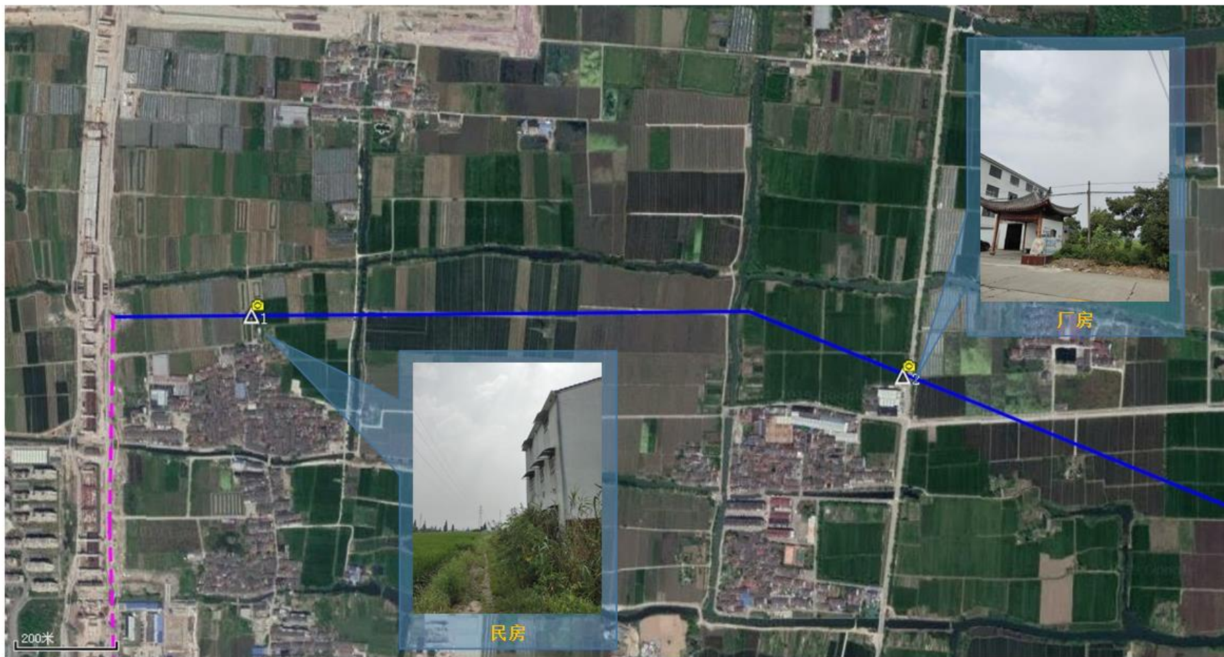
附图 3-2 (a) 蔡郎 110kv 送出工程▲ 1~▲ 2 检测点位示意图
