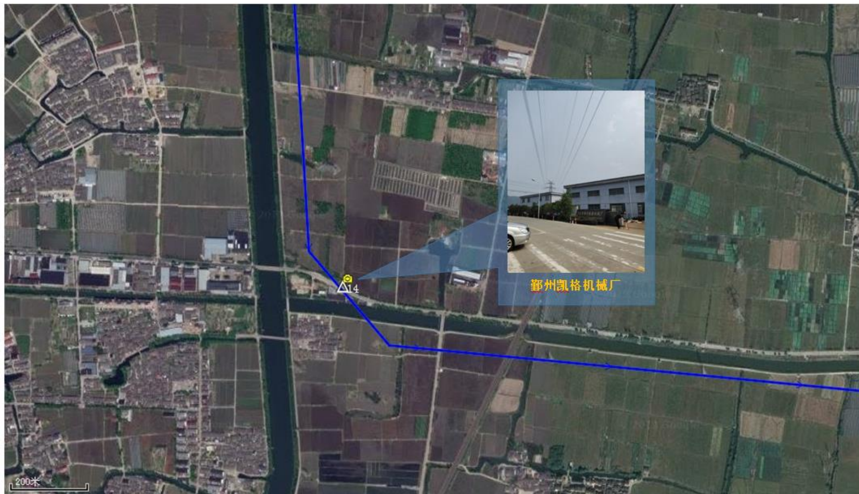
附图 3-3 (j) 220kV 天一~芦江输电线路工程▲14 检测点位示意图检测点位示意图
