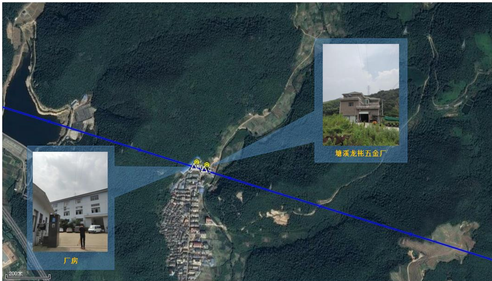
附图 3-3 (f) 220kV 天一~芦江输电线路工程▲ 9~▲ 10 检测点位示意图检测点位示意图
