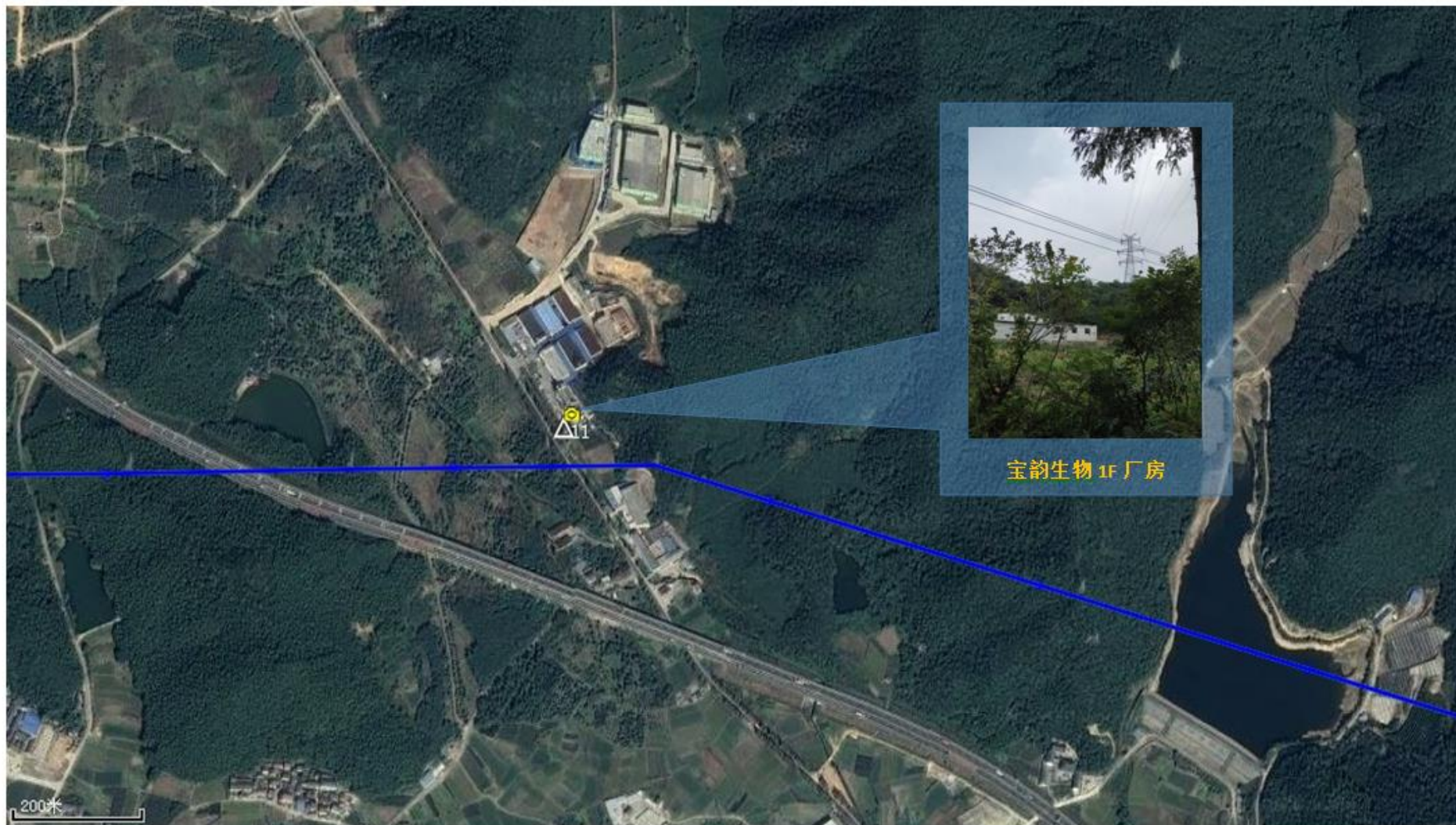
附图 3-3 (g) 220kV 天一~芦江输电线路工程▲ 11 检测点位示意图检测点位示意图
